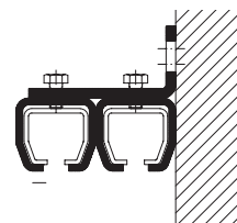
Doppel-Wandmuffe Nr. 301-501 D
