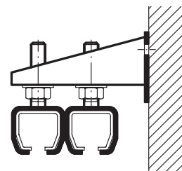
Doppel-Winkelbefestigung Nr. 404 WD / 604 WD / 704 WD
