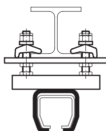
Höhenverstellbare Aufhängekombination Nr. 1309-1709
