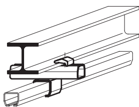
Aufhängekombination Nr. 1302-1702 Ausführung "A"
