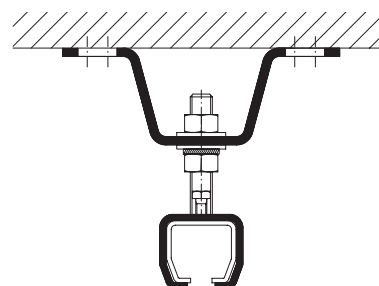
Höhenverstellbare Muffe Nr. 404
